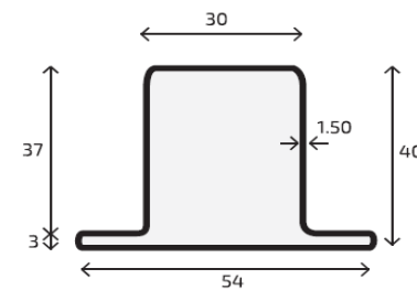
PDS - 41 Peso: 2.053 Kg/m
