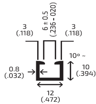
R: 5492 Peso: 0.210 Kg/m
