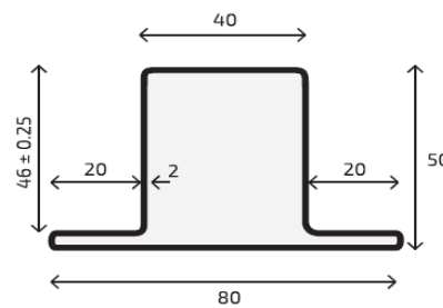
R: 5860 Peso: 3.846 Kg/m
