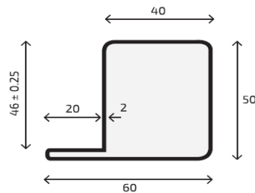
R: 5858 Peso: 3.234 Kg/m
