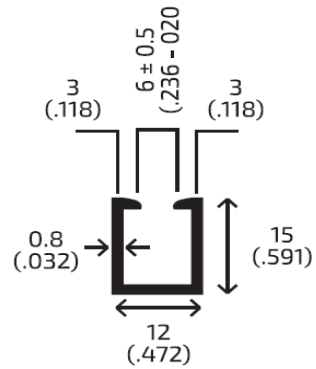
R: 5518 Peso: 0.270 Kg/m
