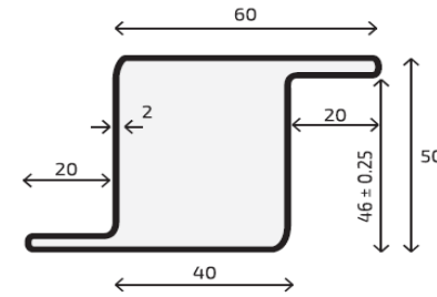
R: 5859 Peso: 3.846 Kg/m
