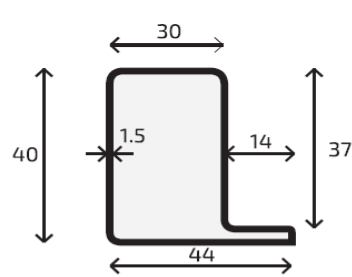
P. Aleta N°1 (PDS 26)
